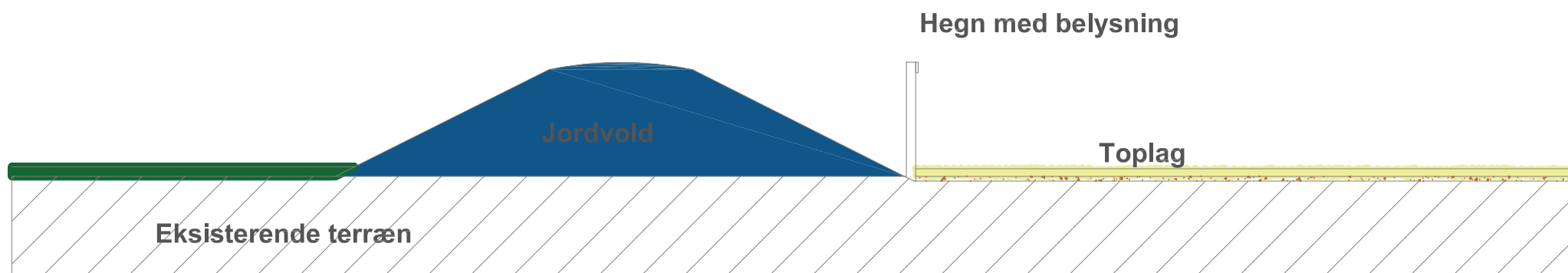
Principsnit
